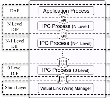
Fig. 2. RINA node
